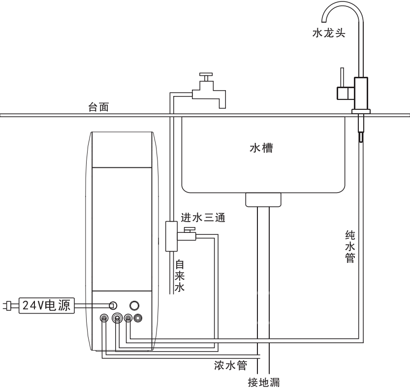
净水机安装示意图
