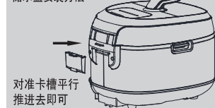
储水箱安装方法
