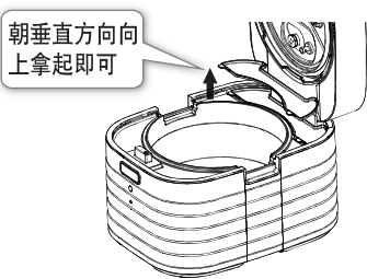
储水盒的拆卸方法
