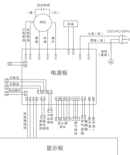
集成灶部分电气原理图
